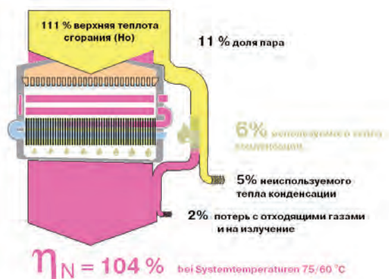
Рис.5: КПД современного конденсационного котла при работе в системе отопления 75/60 °C.
